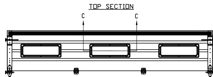
OPTIONAL GLAZED SECTION W/ 24' X 8' WINDOWS N.T.S.
